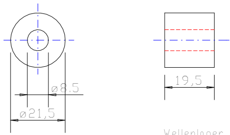
Wellenlager aus P6
